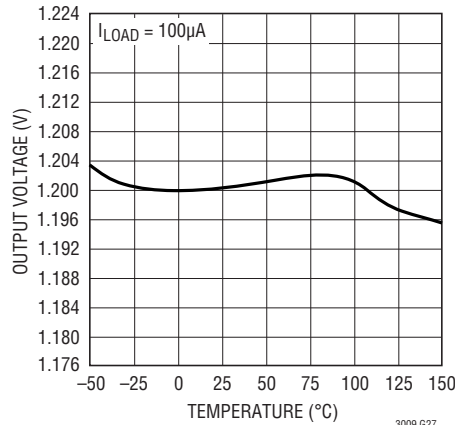
Output Voltage LT3009-1.2
